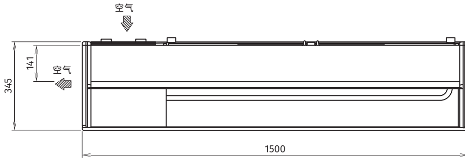
俯视图
